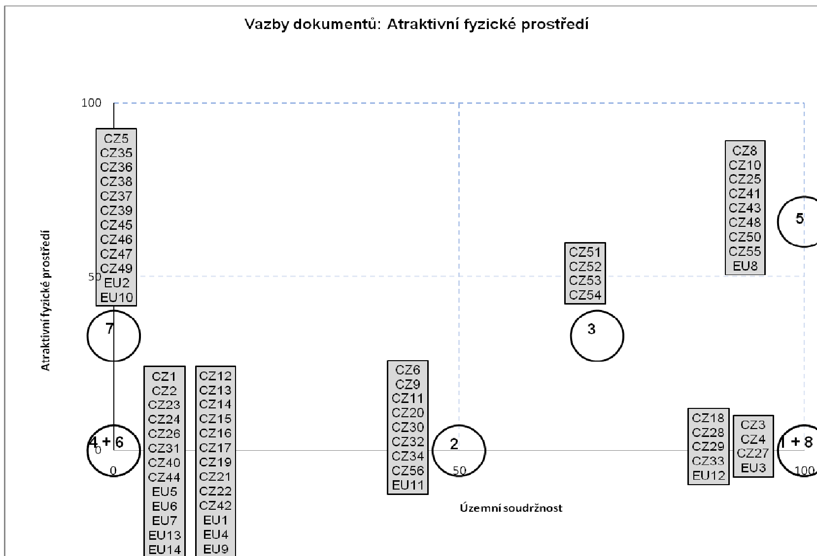
Graf 3: Atraktivní fyzické prostředí a územní soudržnost
