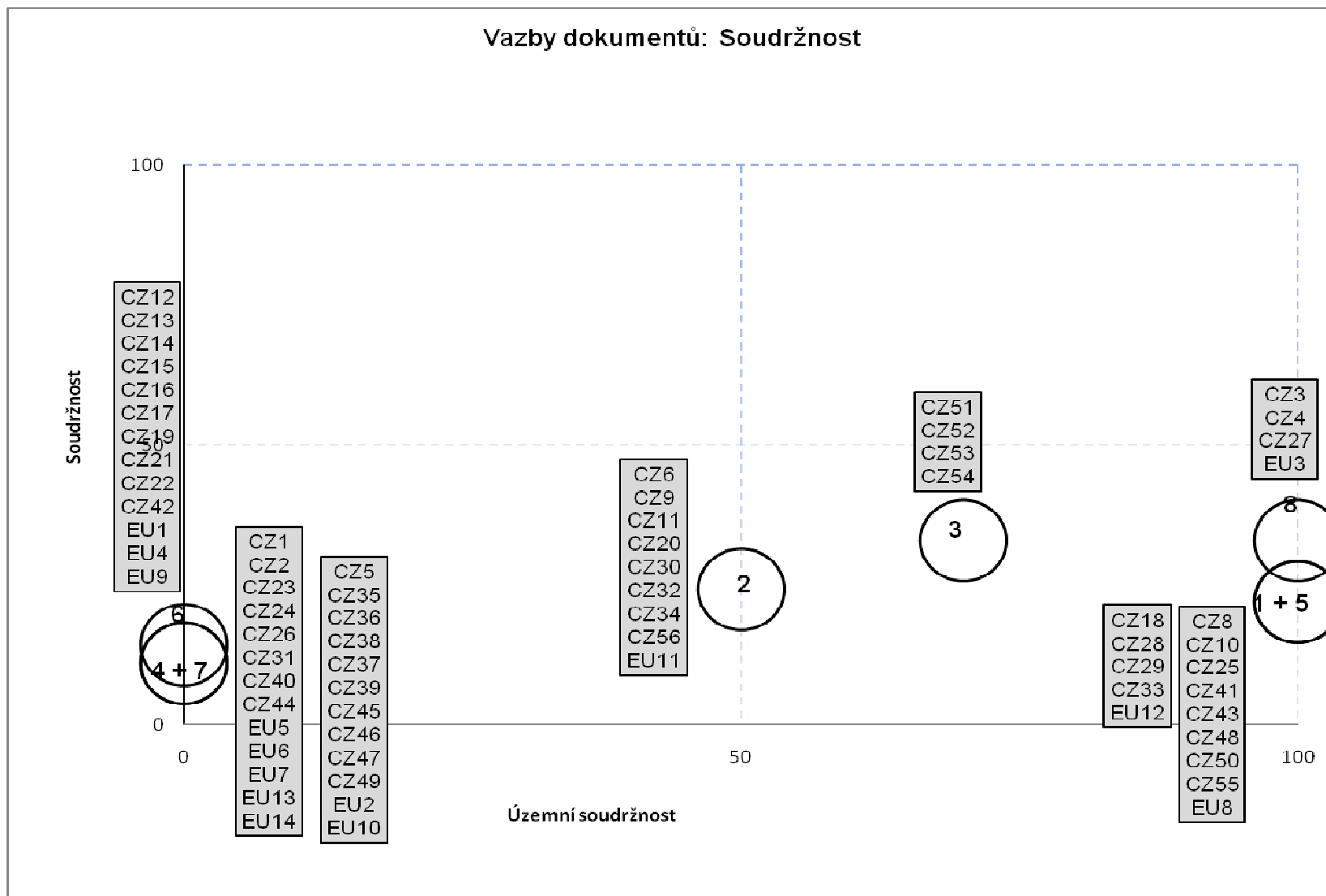
Graf 4: Územní soudržnost a souhrn ostatních pilířů soudržnosti
