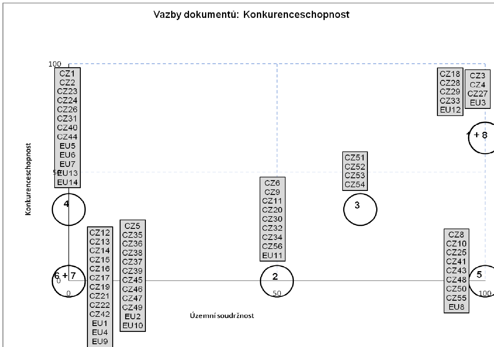
Graf 1: Konkurenceschopnost a územní soudržnost
