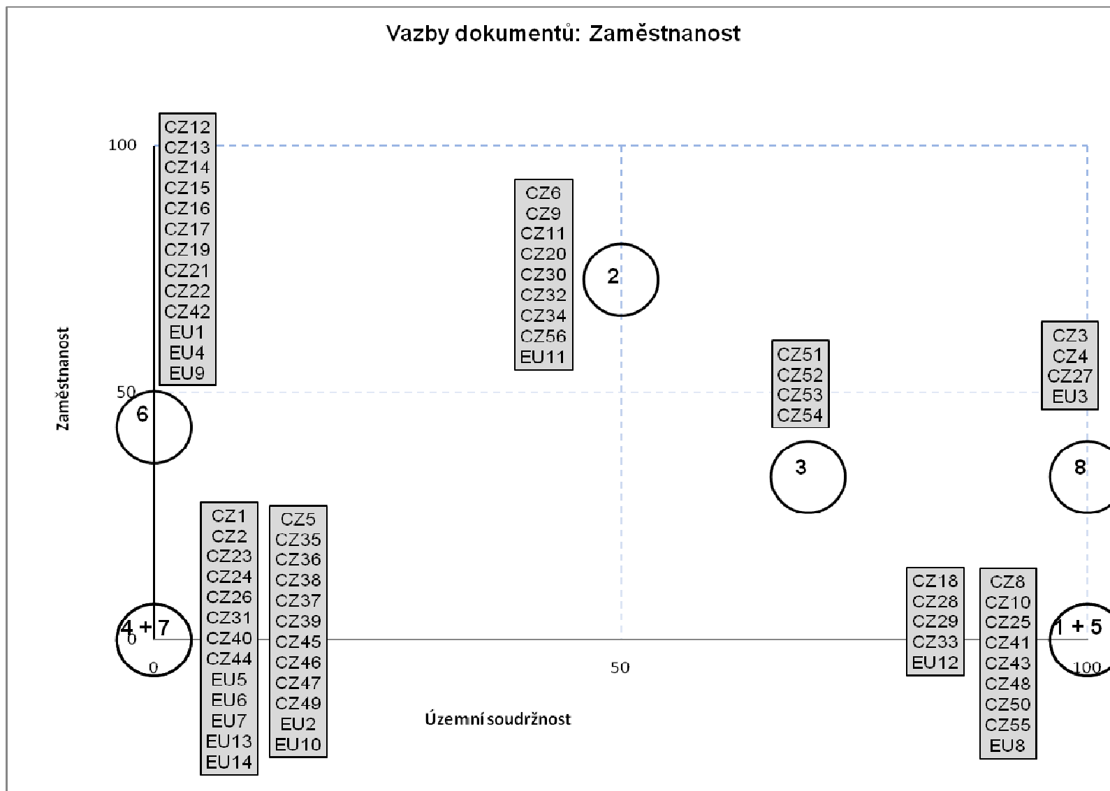
Graf 2: Zaměstnanost a územní soudržnost
